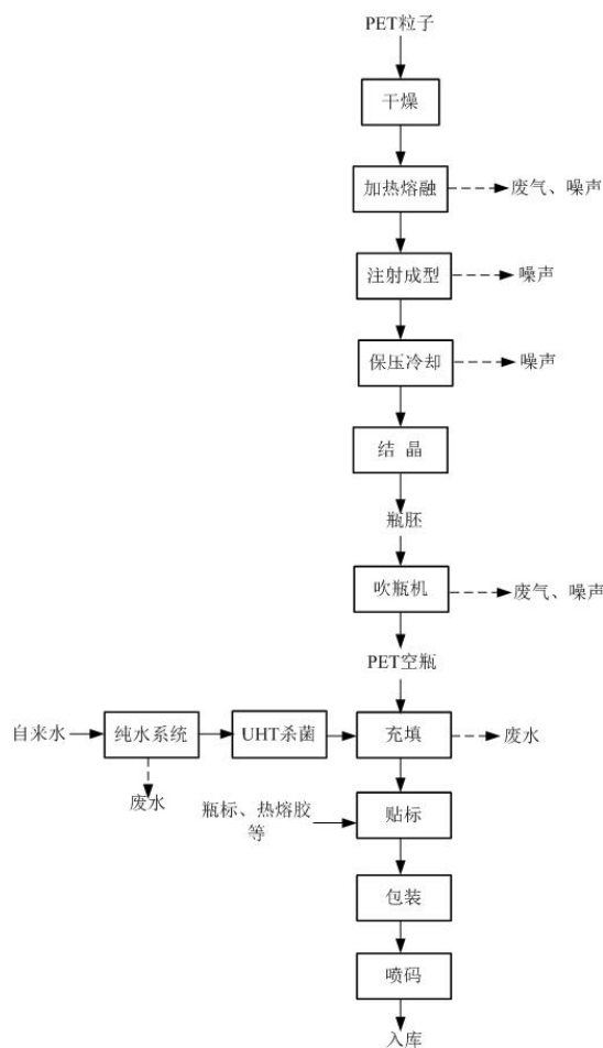
图 2-1 本项目生产工艺流程图
