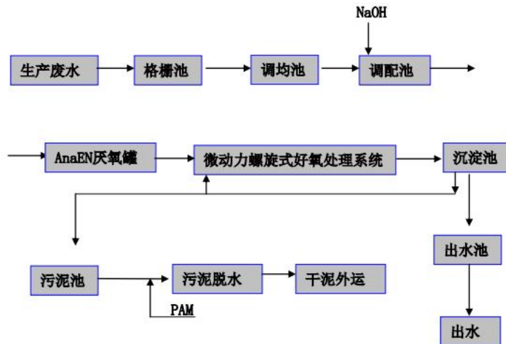
图 3-1 企业废水处理工艺流程图
